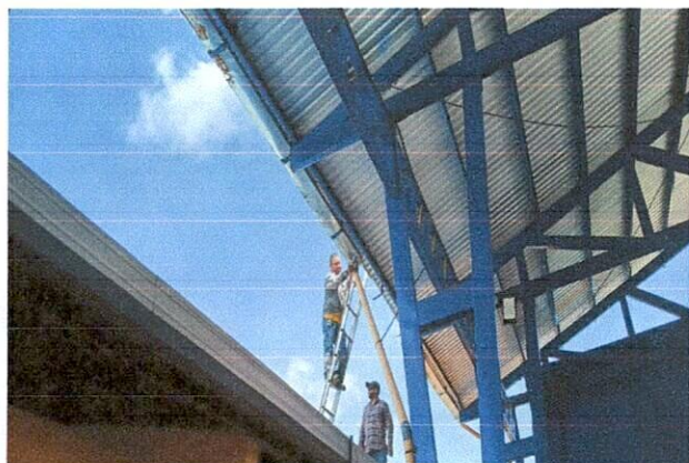
Foto 3: Instalación de canales pluviales
